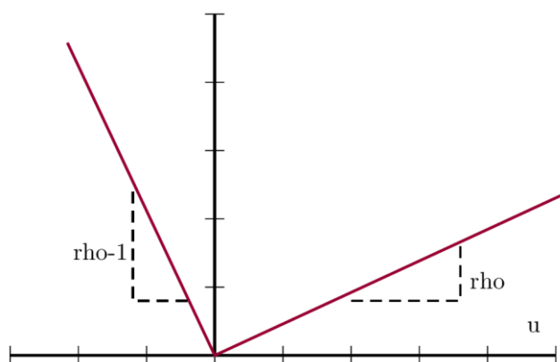
Figura A1 : Funzione \rho_q
